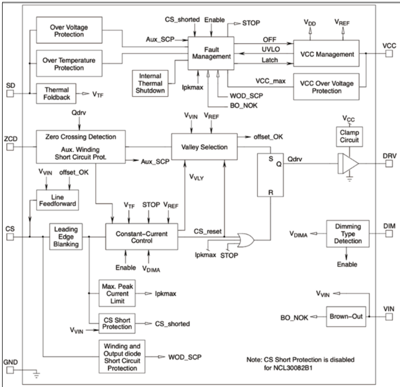
圖 1：NCL30082 內部電路結構
